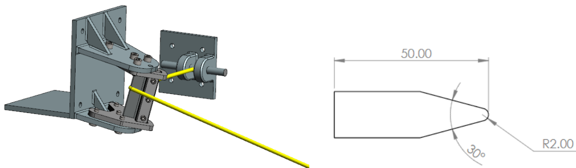
Figure A2 – Configuration générale de l'essai de traction et détail de la lame
