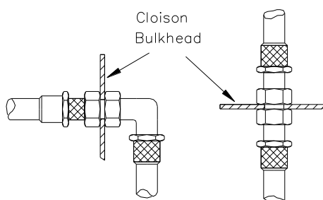
Dessin / Drawing 253-59
