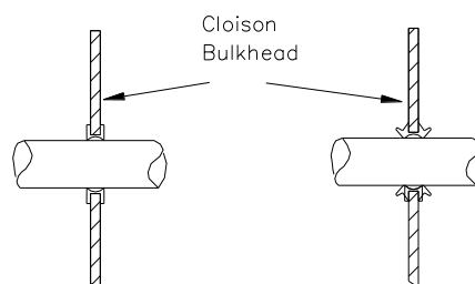
Dessin / Drawing 253-60
