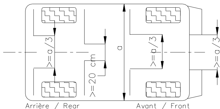
Dessin / Drawing 252-6
