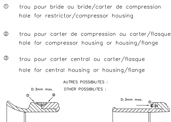
Dessin / Drawing 254-4
