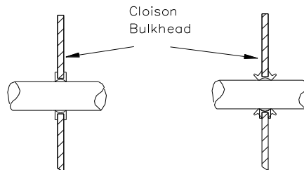
Dessin / Drawing 253-60
