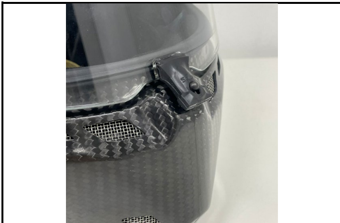
D1) Vue du mécanisme de verrouillage en position de visière fermée / View of the locking mechanism in closed visor position
