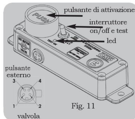
Fig 11: centralina di comando impianto e dettaglio del pin-out connettore:
