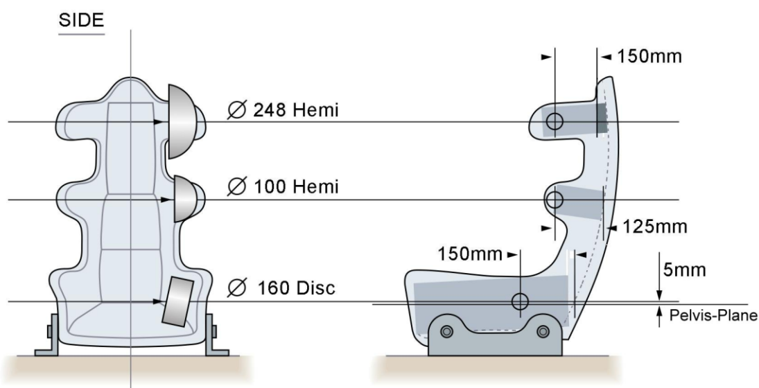
Figure B1. Configuration d'essai pour l'application d'une charge dans la direction latérale
