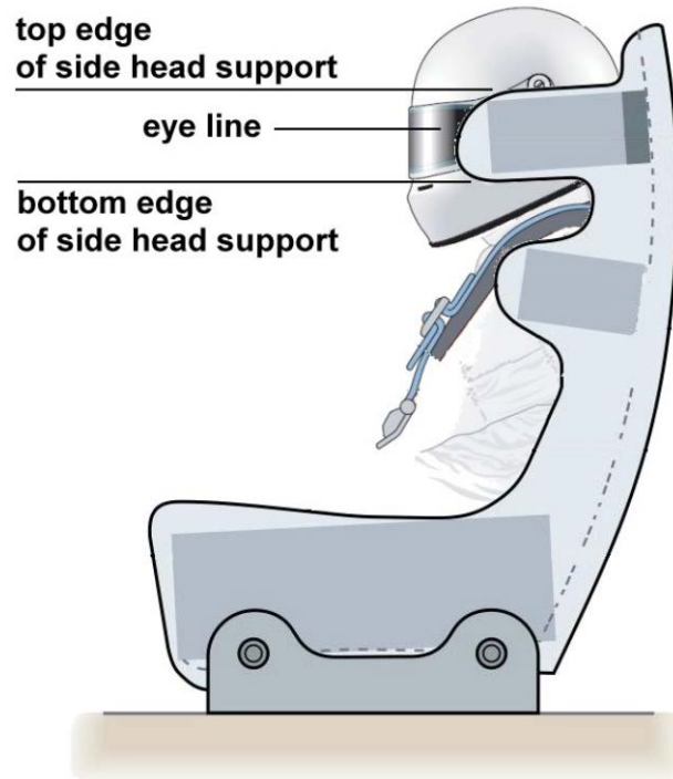
Figure 2. Position recommandée pour la tête des pilotes par rapport au support latéral de la tête Figure 2. Recommended position of drivers head relative to side head support
