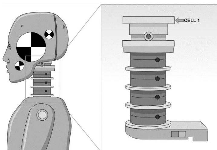
Figure A7 – Montage du capteur de force Figure A7 – Load cell assembly
