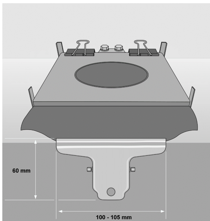
Figure A-3.3 Dimensions de la pince à dessin Figure A-3.3 Dimensions of the bulldog clip
