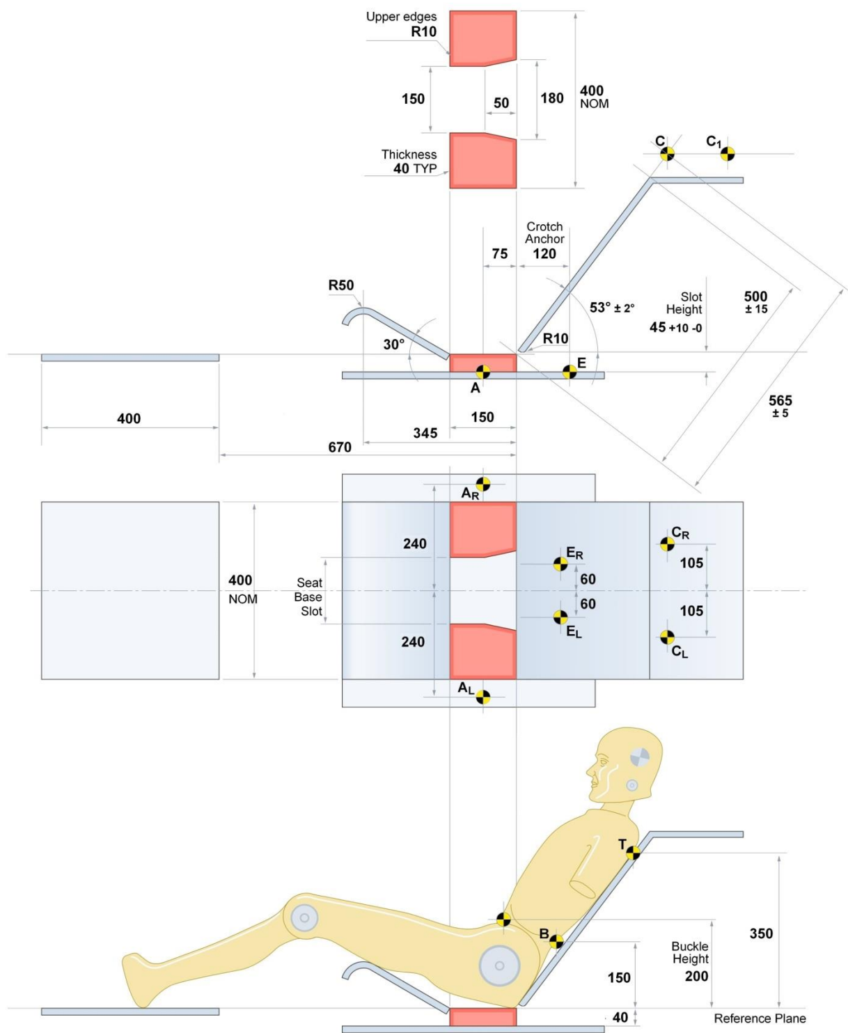
Figure B 1. Descriptif du siège, du chariot et des ancrages (dimensions en millimètres - la tolérance pour les points de mesure est de ± 5 mm )
