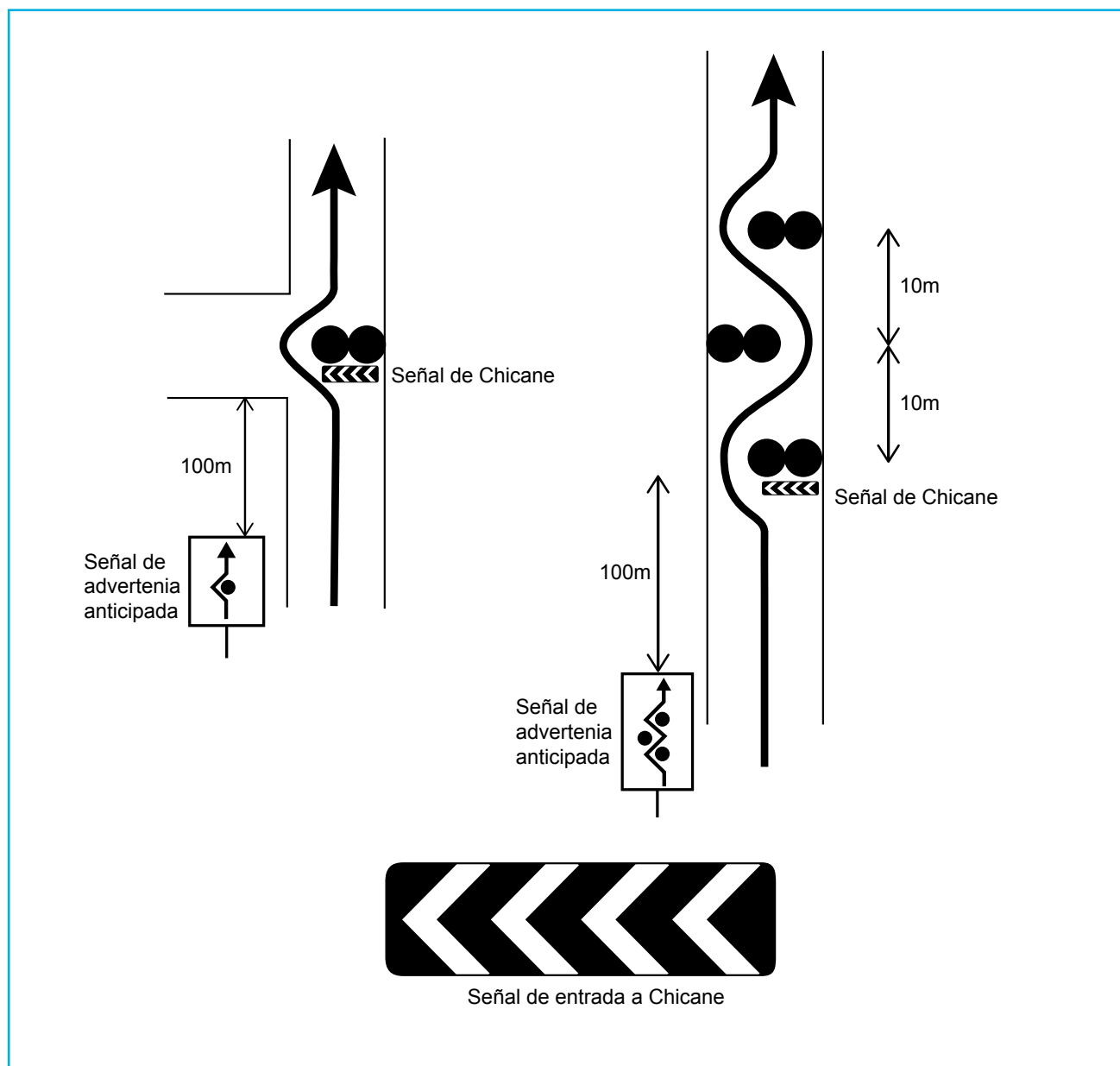
Perfil de chicane recomendado
