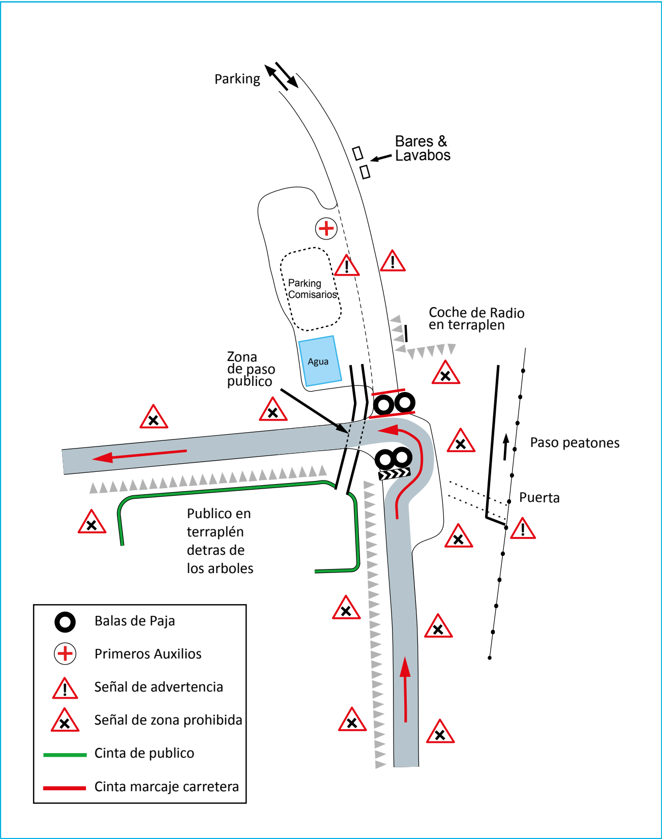
MAPA DE TRAMO ESPECIAL DETALLADO PARA PLAN DE SEGURIDAD
