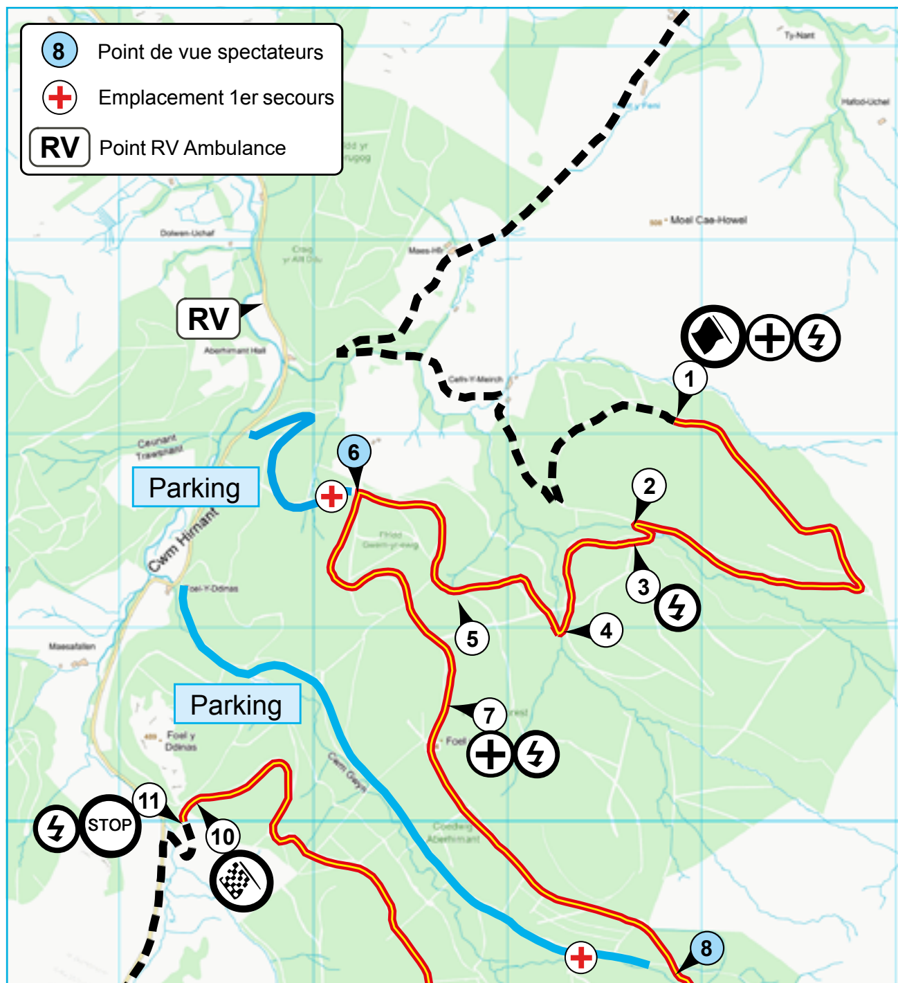
Carte détaillée de spéciale pour le plan de sécurité
