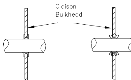
Dessin / Drawing 253-60
