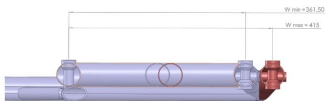
Dessin/Drawing 279E-15
