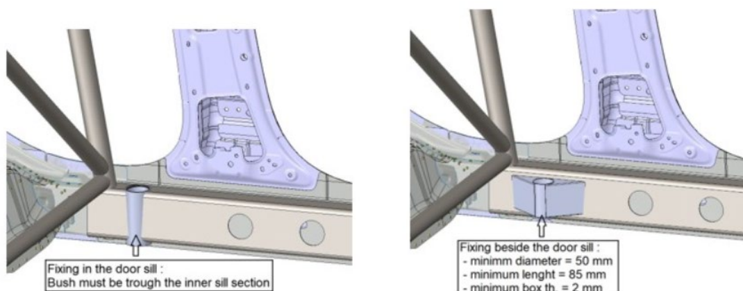
Dessin/Drawing 279E-13
