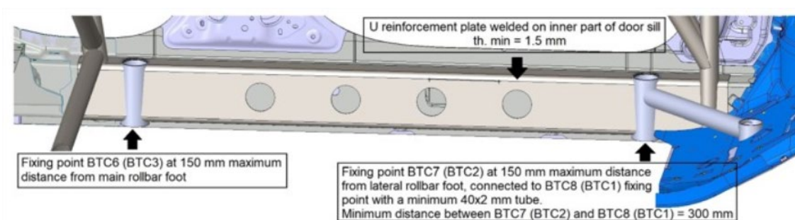
Dessin/Drawing 279E-15
