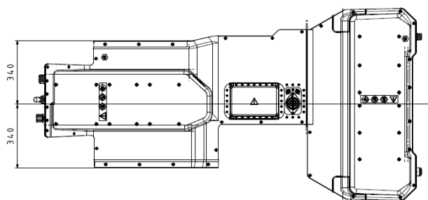
Dessin/Drawing 279E-11
