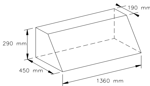
Dessin / Drawing 279-4
