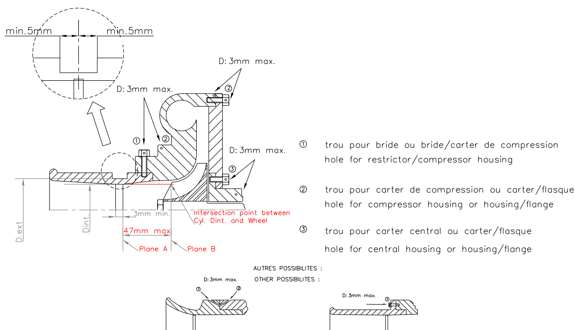
Dessin / Drawing 254-4
