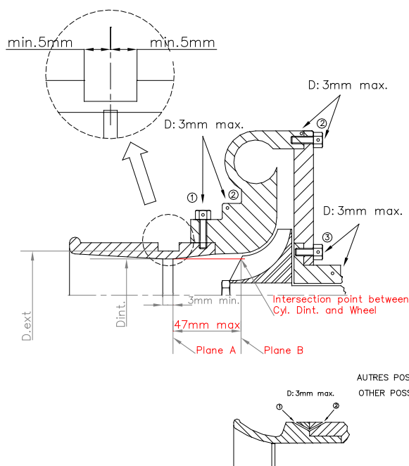
Dessin / Drawing 254-4
