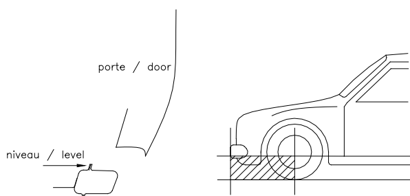
Dessin / Drawing 279-3
