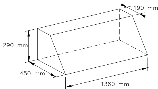
Dessin / Drawing 279-4
