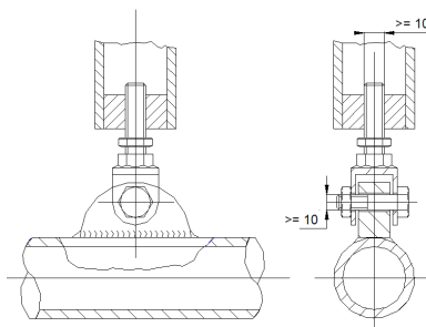
Dessin/Drawing SC-DJ-9
