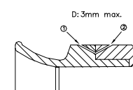
Dessin / Drawing 254-4
