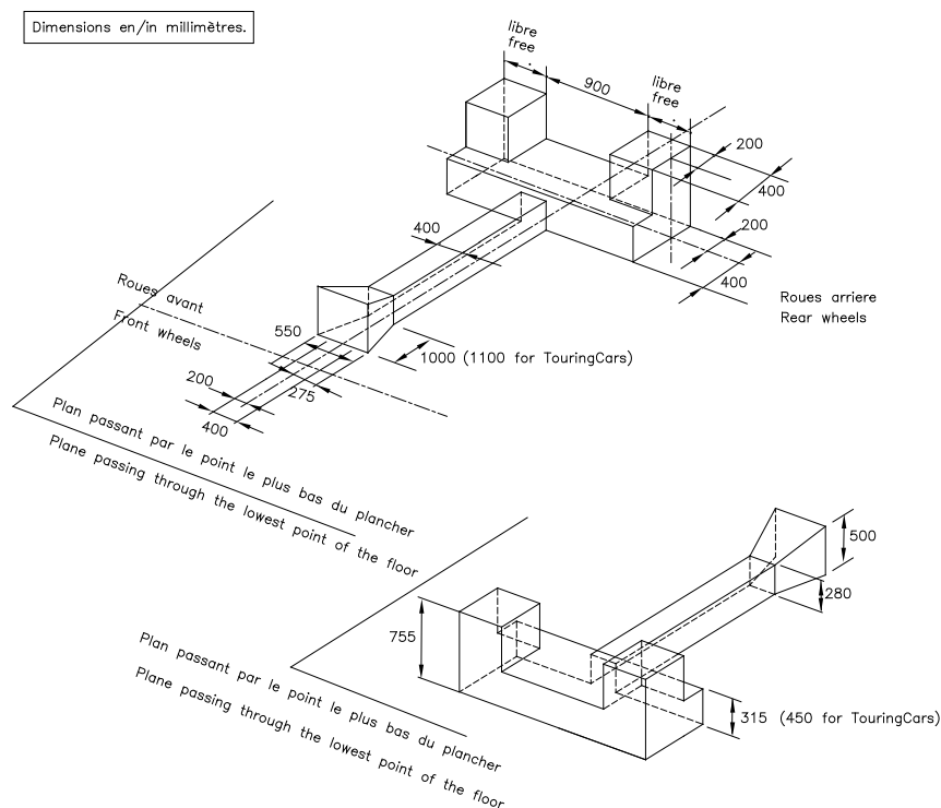
Dessin / Drawing 279-1
