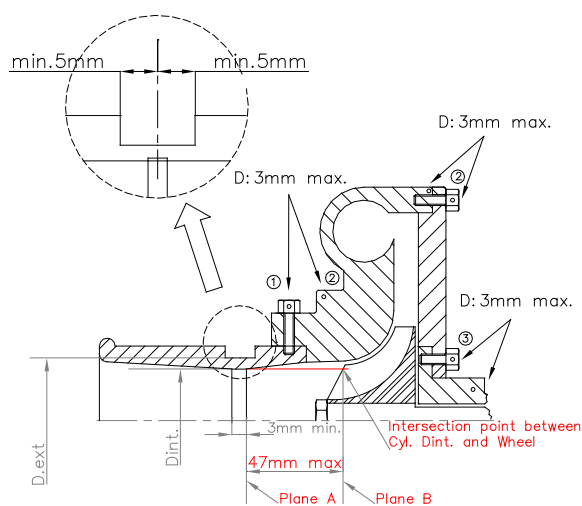
Dessin / Drawing 254-4
