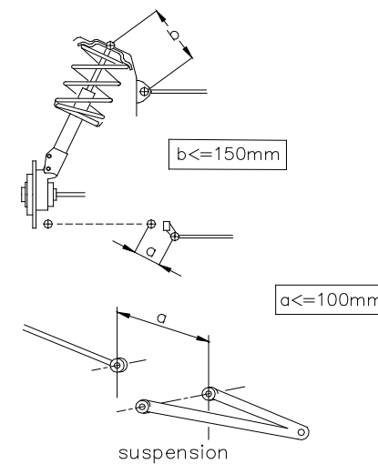
Dessin / Drawing 255-4
