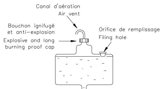
Dessin / Drawing 252-4
