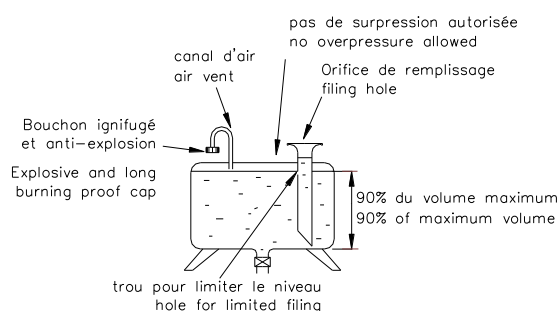
Dessin / Drawing 252-3
