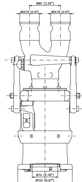
Parallèle / Parallel
