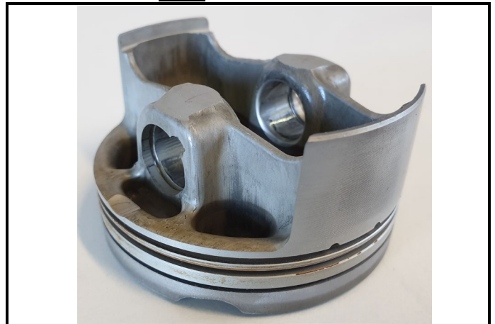
C4-2) Piston de \frac{3}{4} dessous Piston from \frac{3}{4} bottom
