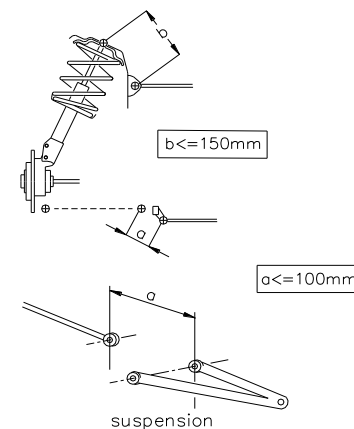
Dessin / Drawing 255-4
