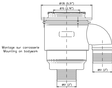
Accoupler femelle
