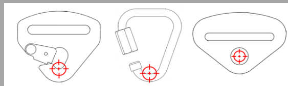
Exemples de points de rotation de l'ancrage de sangle Examples of pivot points of the anchorage of the strap
