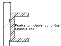
120mm max. à l'extérieur de la poutre principale du châssis 120mm max. from the outer surface of the chassis rail
